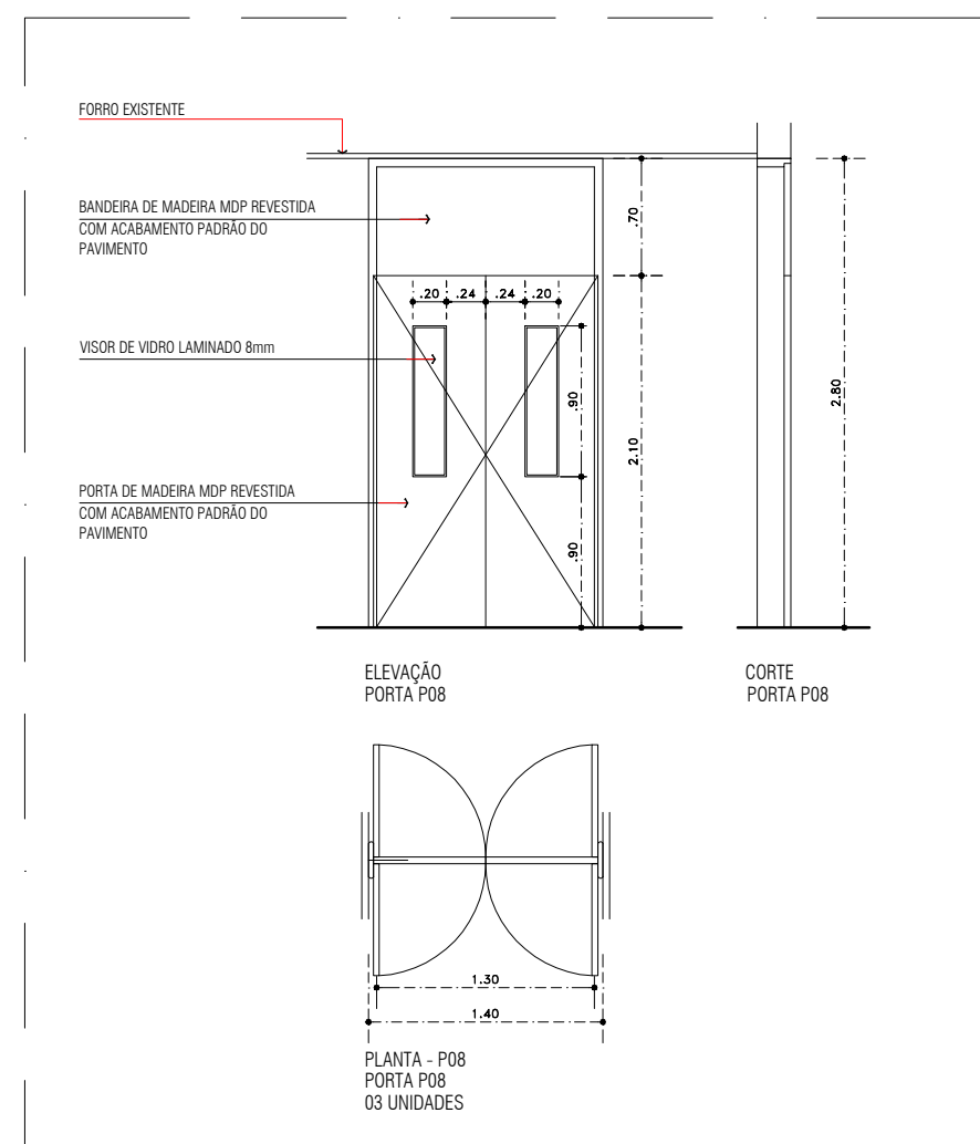
DET. PORTA P08 ESCALA 1/50
