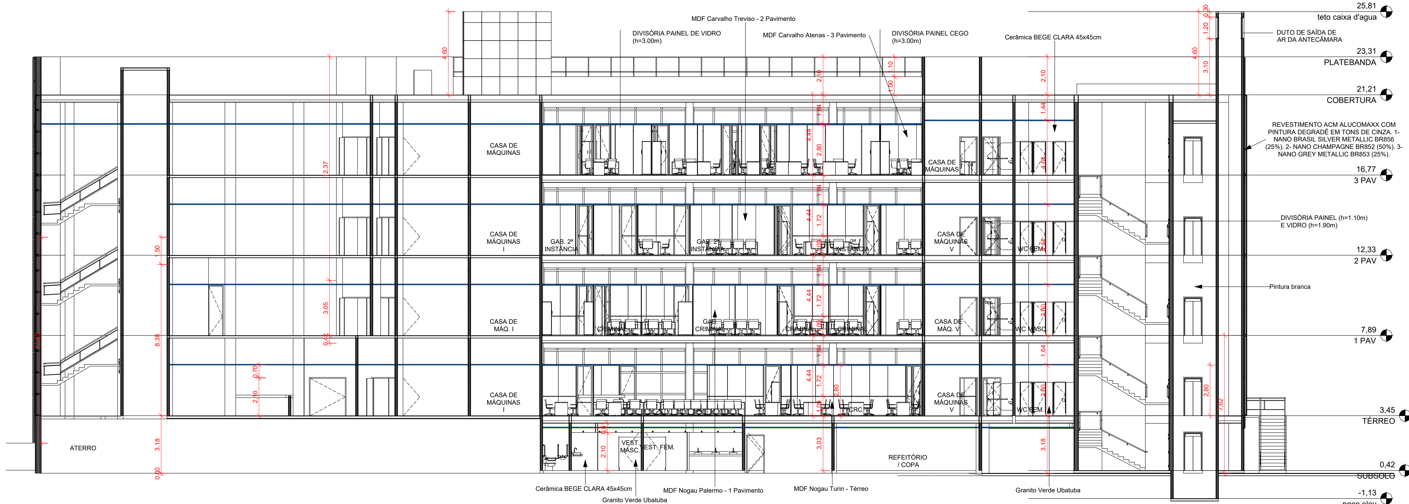
2 CORTE BB' ESCALA 1:125
