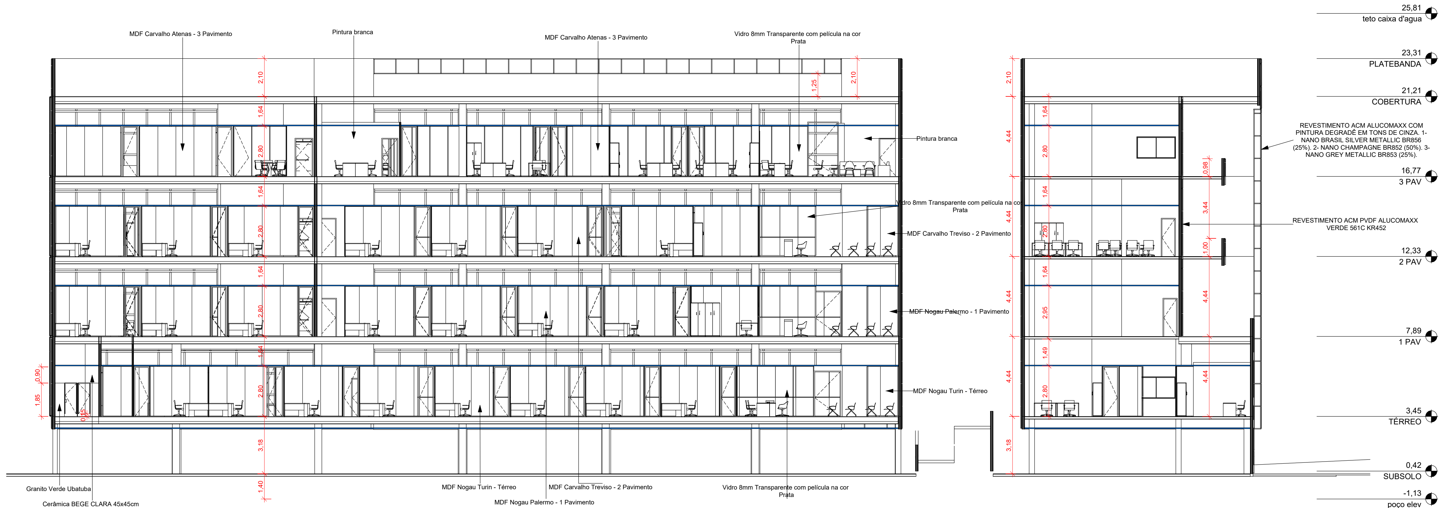
1 CORTE AA' ESCALA 1:125
