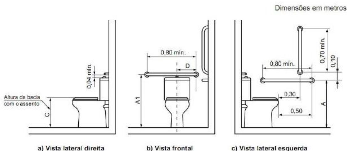
Referência barra de apoio
