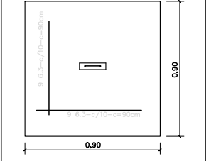
DETALHE AÇO TAMPA: S/ESC.
