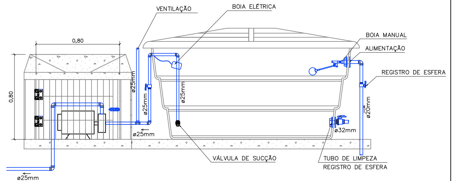
02 DETALHAMENTO: RESERVATORIO INFERIOR ESCALA _____ S/ESCALA
