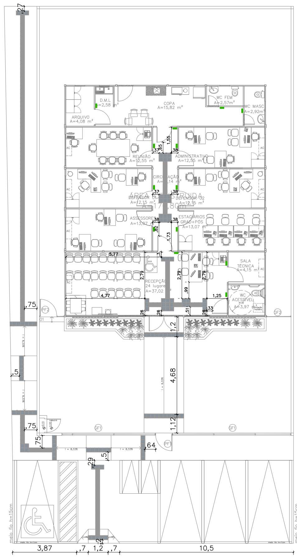
01 SINALIZAÇÃO TÁTIL- INTERNA E EXTERNA ESCALA 1/100
