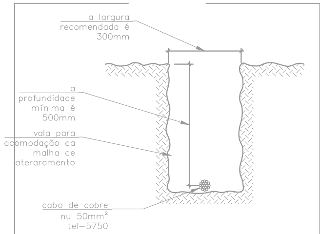
03 DET 02: VALA DE MALHA DE ATERAMENTO SEM ESCALA
