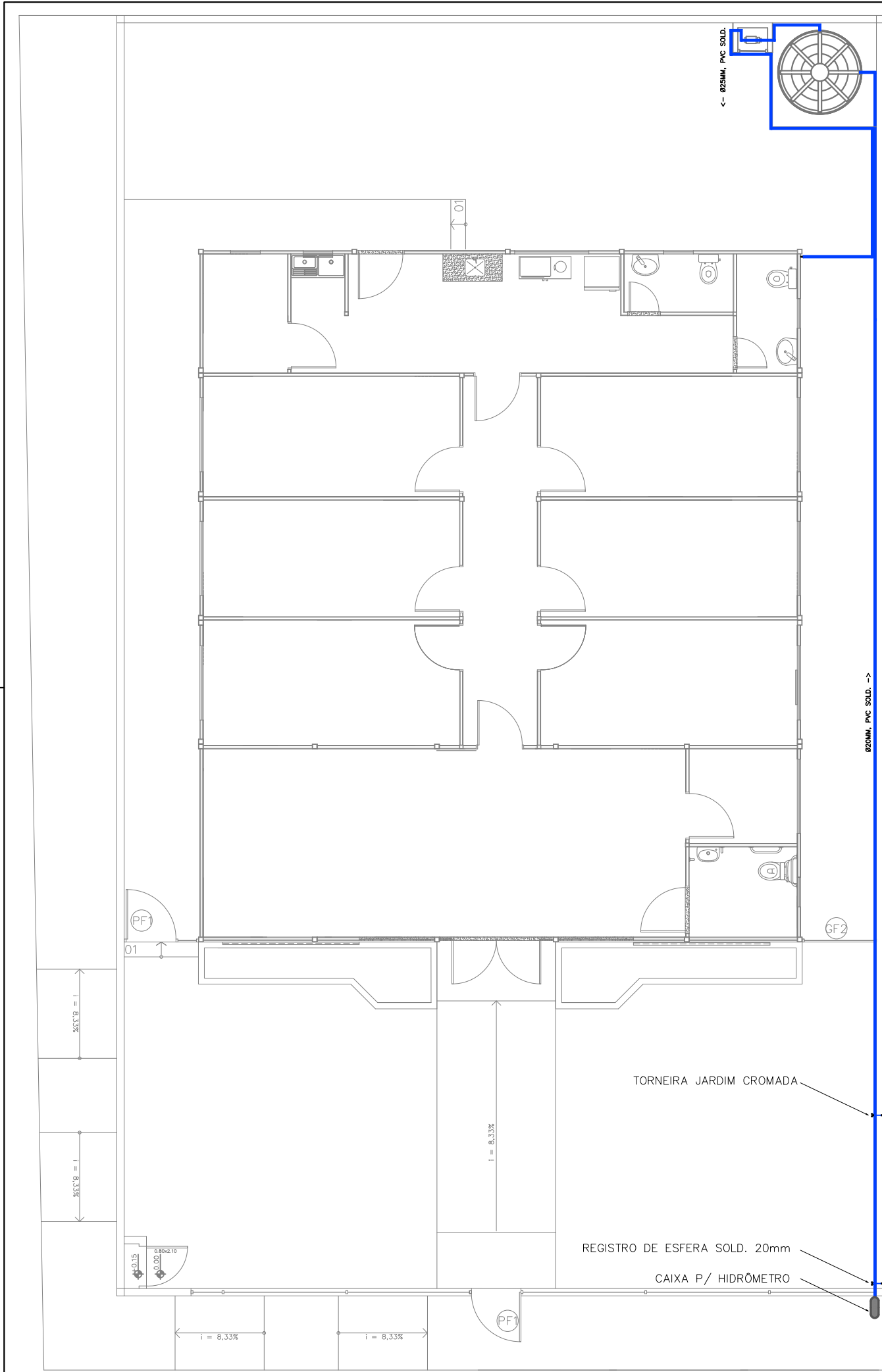
01 ABASTECIMENTO DE ÁGUA ESCALA _____ 1/100
