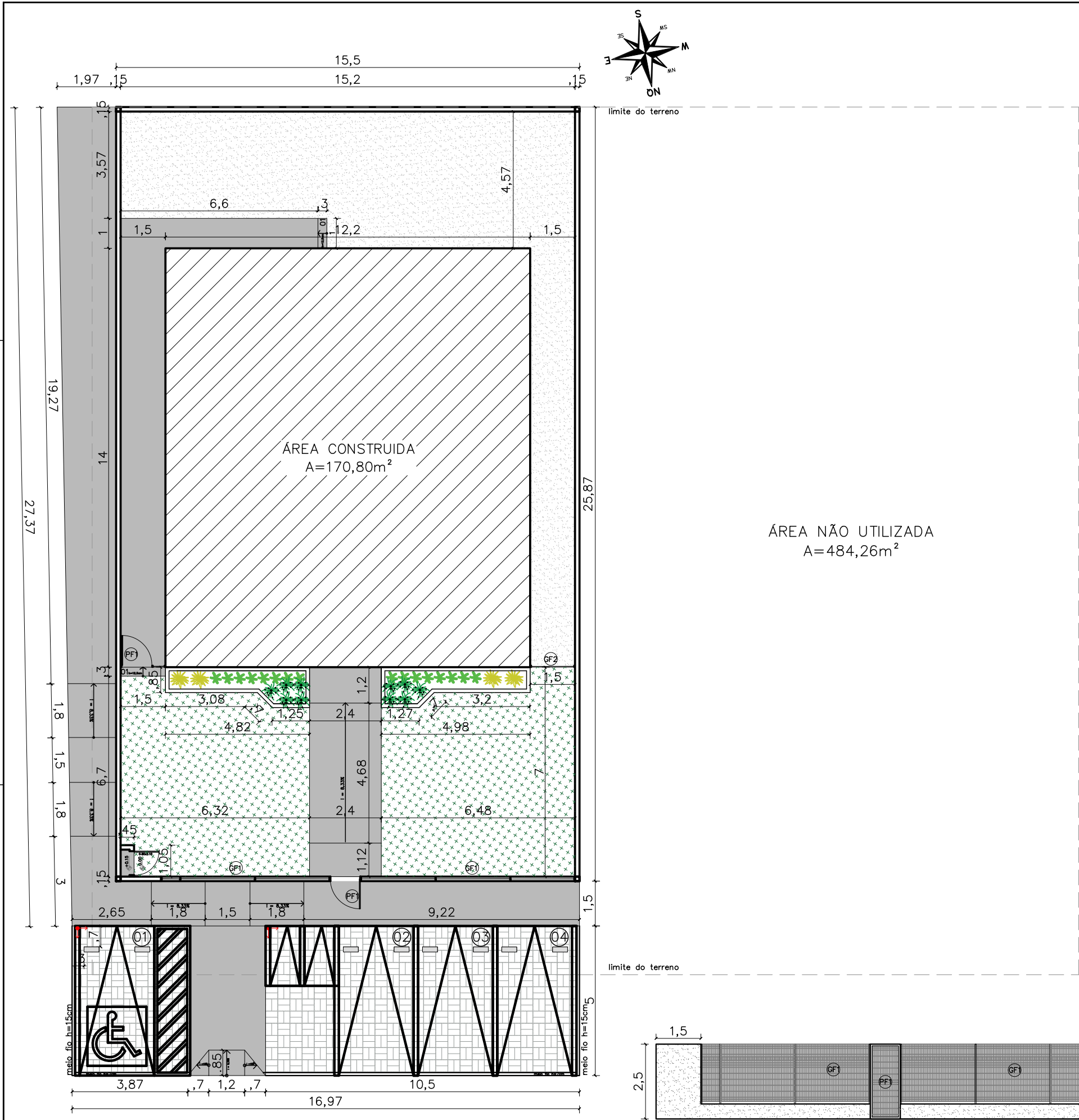
01 IMPLANTAÇÃO ESCALA 1/100
